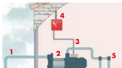
Circuit jardin avec vanne manuelle
