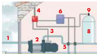
Circuit usage domestique et jardin
